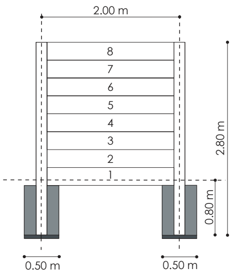
8 placas: 2,08 m
