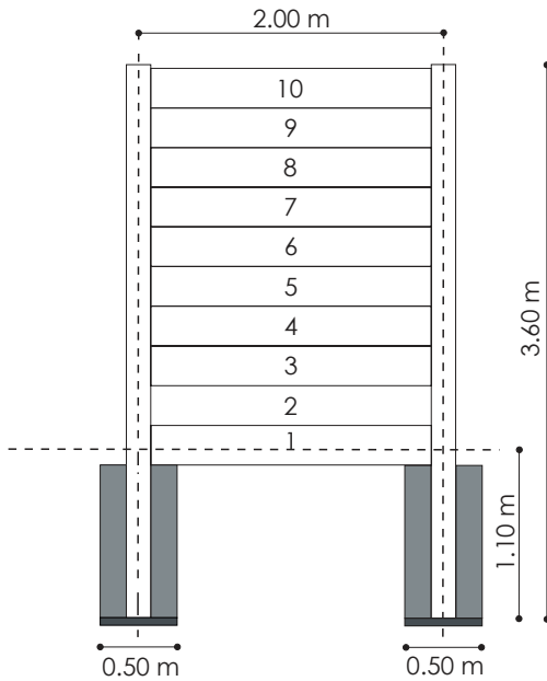
10 placas: 2,60 m
